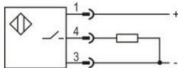
PNP NO
