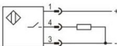
PNP NO
