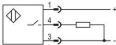
PNP NO
