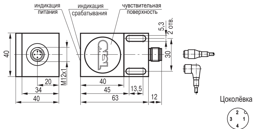
Габаритный чертеж
