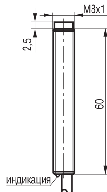
Габаритный чертеж
