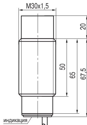
Габаритный чертеж
