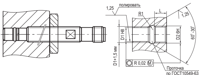
Схема монтажа
