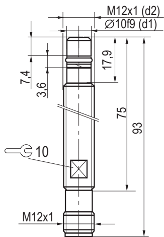
Габаритный чертеж
