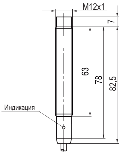
Габаритный чертёж
