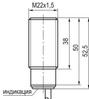
Габаритный чертеж
