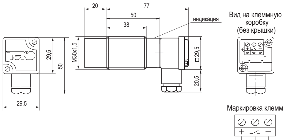
Габаритный чертеж
