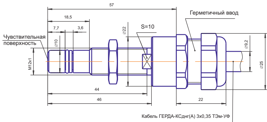
Габаритный чертеж
