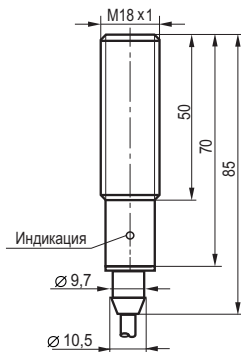
Габаритный чертеж
