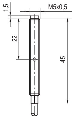
Габаритный чертеж
