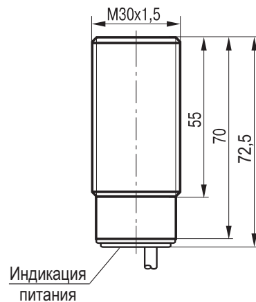
Габаритный чертеж
