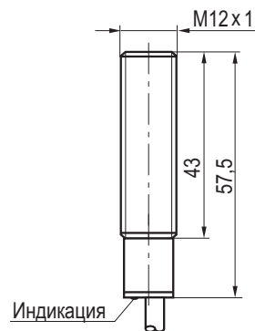
Габаритный чертеж
