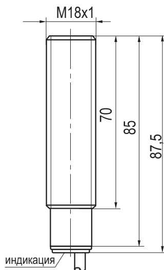
Габаритный чертеж
