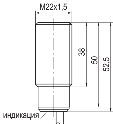
Габаритный чертеж
