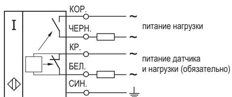
Схема подключения
