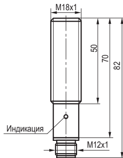
Габаритный чертеж
