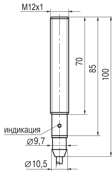
Габаритный чертеж
