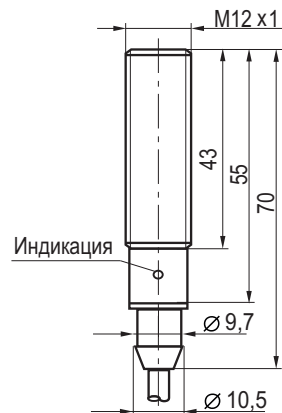
Габаритный чертеж
