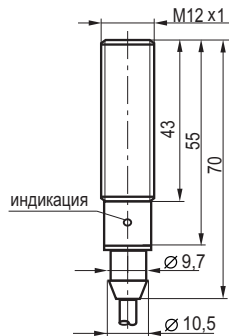
Габаритный чертеж
