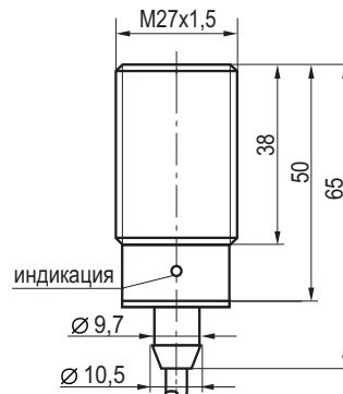
Габаритный чертеж
