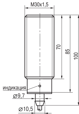
Габаритный чертёж
