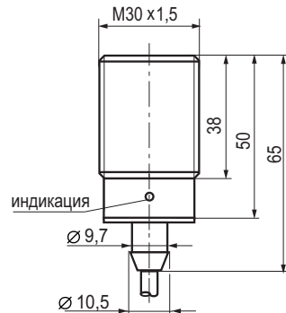
Габаритный чертеж
