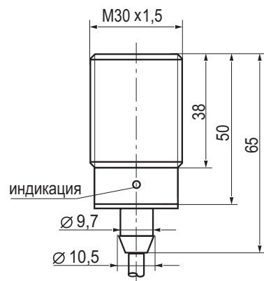
Габаритный чертеж
