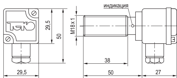
Габаритный чертеж
