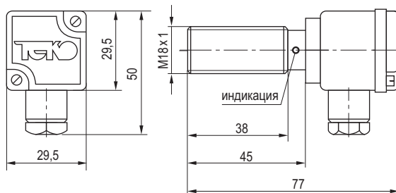
Габаритный чертеж
