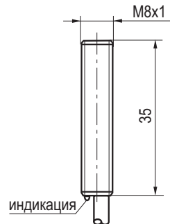
Габаритный чертеж
