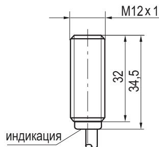
Габаритный чертеж
