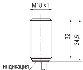
Габаритный чертеж
