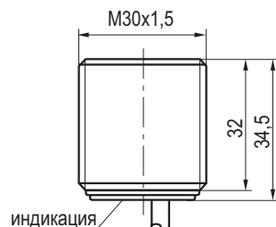
Габаритный чертеж
