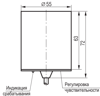
Габаритный чертеж
