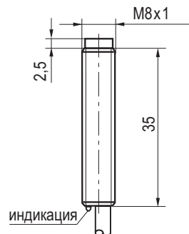
Габаритный чертеж
