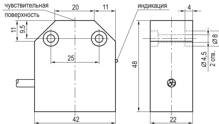
Габаритный чертеж
