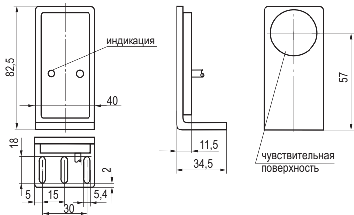
Габаритный чертеж
