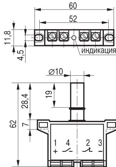
Габаритный чертеж
