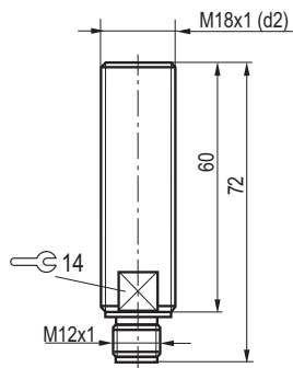
Габаритный чертеж
