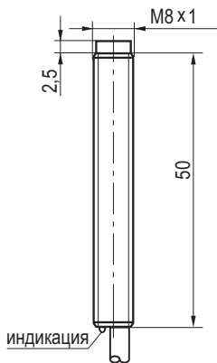
Габаритный чертеж
