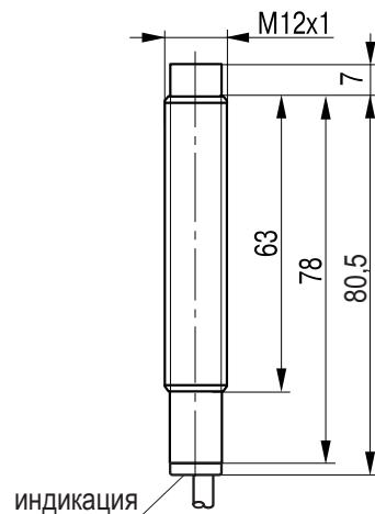
Габаритный чертеж
