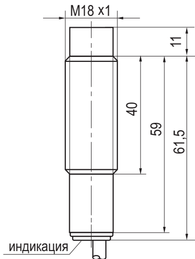
Габаритный чертеж
