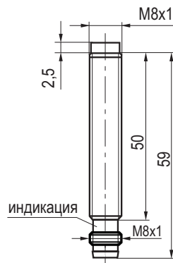
Габаритный чертеж
