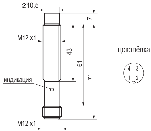
Габаритный чертеж
