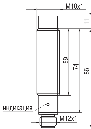
Габаритный чертёж
