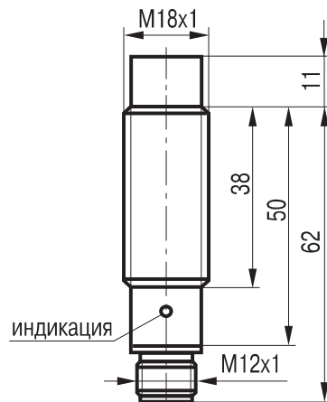
Габаритный чертеж
