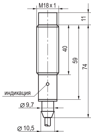
Габаритный чертеж
