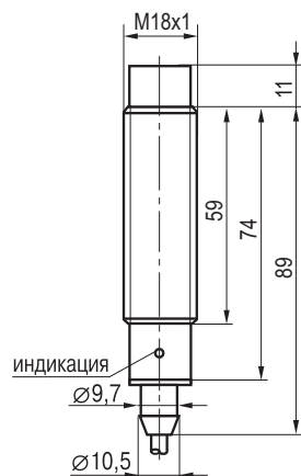
Габаритный чертеж
