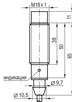
Габаритный чертеж
