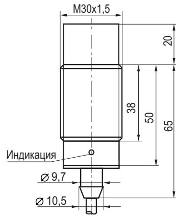
Габаритный чертеж
