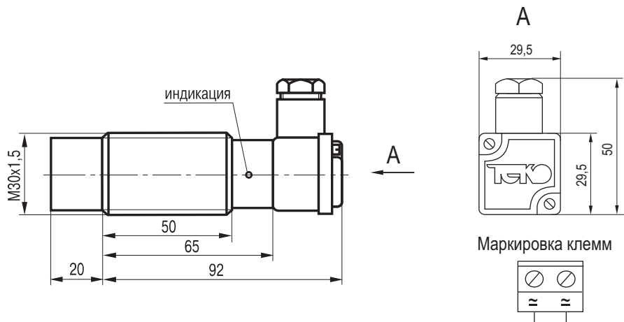
Габаритный чертёж
